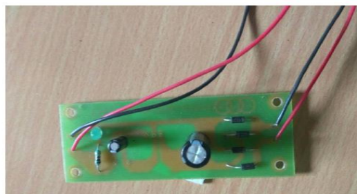
Fig5: Rectifier
